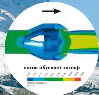
Регулирующий клапан осевого типа Осевое течение и Total Velocity Management® - ключ к надежности
