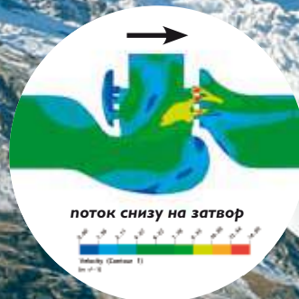
Обычный седельный клапан Разновекторность траекторий потока снижает рабочие характеристики трима и приводит к разбалансировке усилий в нем.
